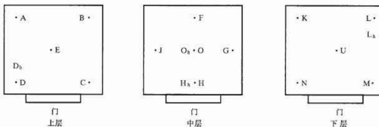
图 2 试验设备容积大于 2\text{ m}^3 时温湿度测量点布放位置
