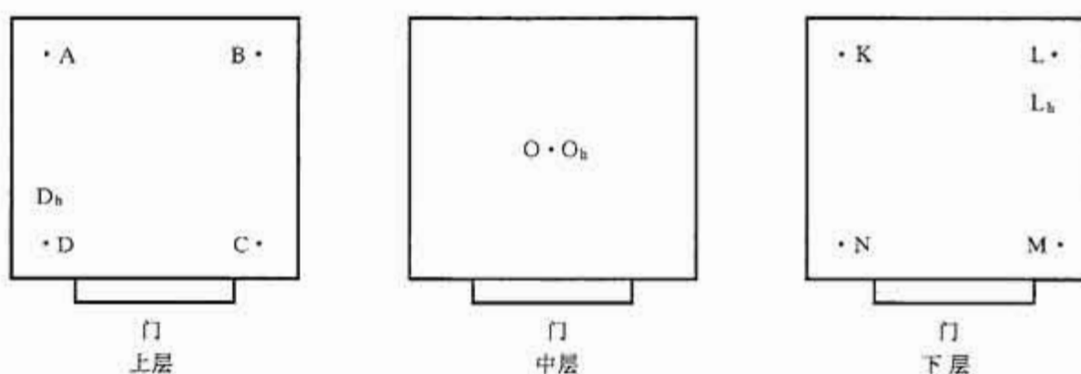
图 1 试验设备容积小于或等于 2\text{ m}^3 时温湿度测量点布放位置
